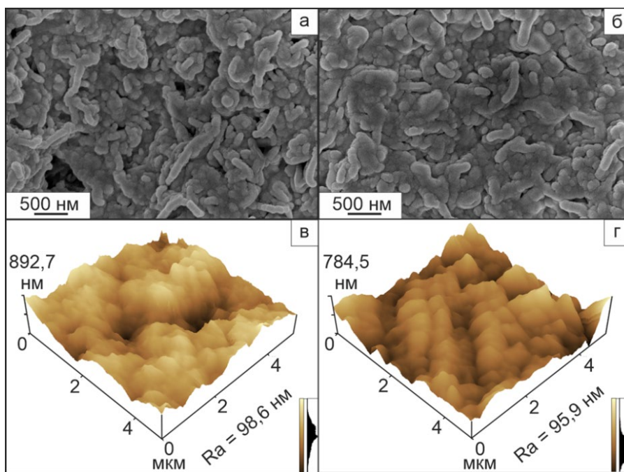
Рисунок 2 – Морфология пленки полимерной системы до (а, в) и после термической активации (б, г). Показаны изменения, фиксируемые СЭМ (а, б) и АСМ (в, г)
