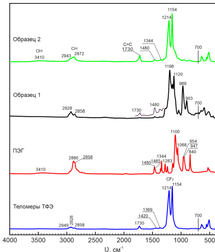
Рисунок 3 – ИК-спектры полимерной системы до и после активации, а также ее отдельных компонентов
