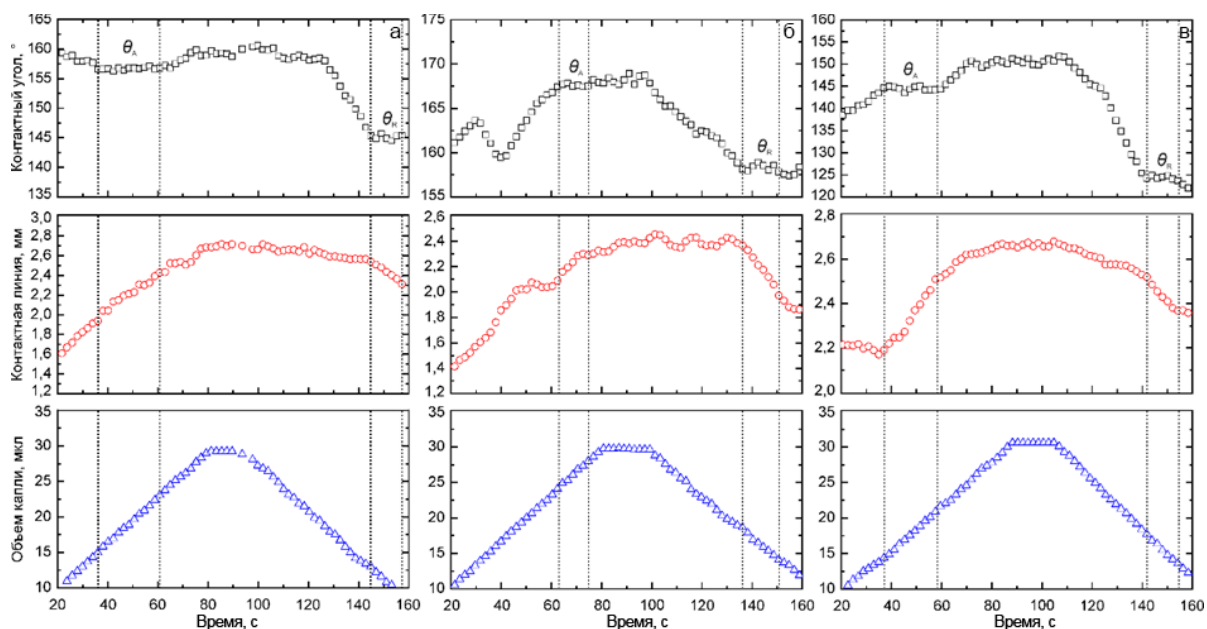
Рисунок 6 – Графики изменения контактного угла (верхняя панель), длины контактной линии (средняя панель) и объема капли (нижняя) в процессе измерения углов натекания и оттекания на поверхности КП 1 (а), КП 2 (б) и КП 3 (в), сформированных на магниевом сплаве МА8
