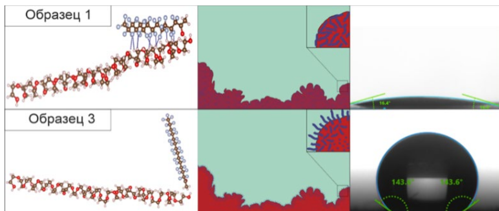
Рисунок 5 – Поведение полимерной системы до и после термического воздействия
