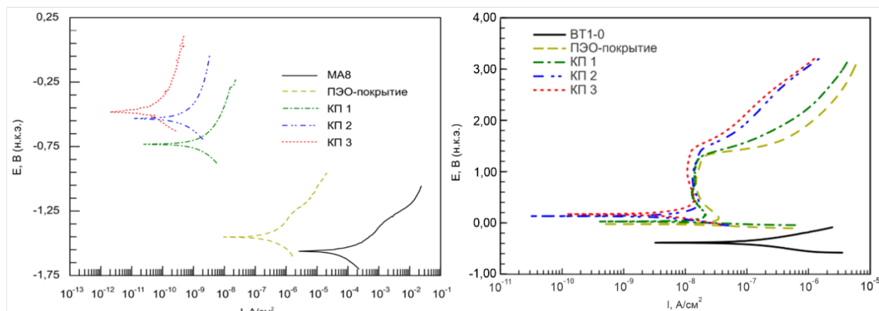
Рисунок 8 – Потенциодинамические поляризационные кривые для образцов из магниевого сплава МА8 и технического титана марки ВТ1-0 с разными видами поверхностной обработки
