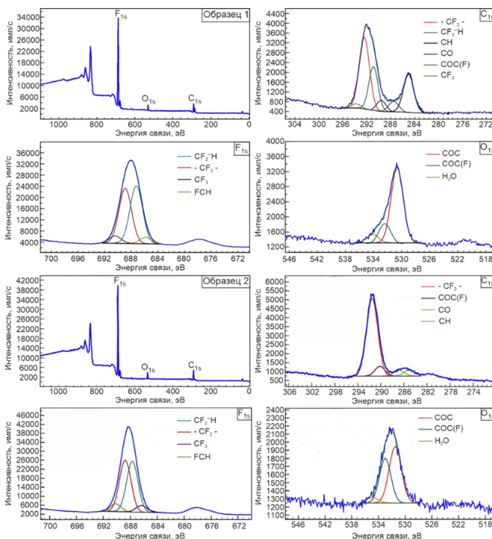
Рисунок 4 – Обзорный спектр и спектры высокого разрешения для образцов 1 и 2 с разложением основных пиков элементов полимерной системы
