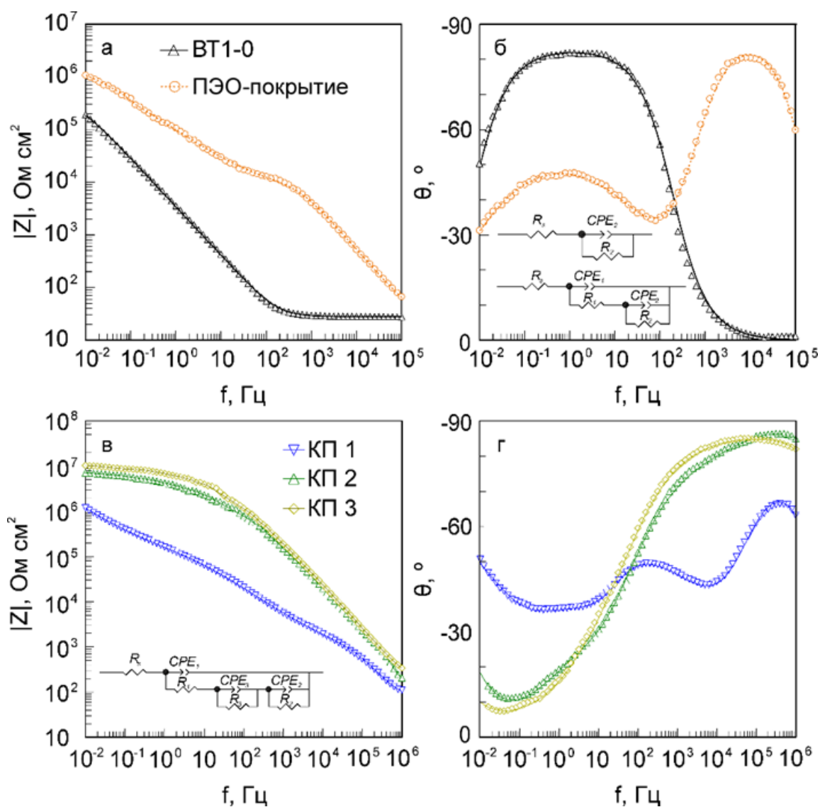
Рисунок 4.14 – Диаграммы Бode для образцов из титана марки VT1-0 без покрытия и с ПЭО-покрытием (а, б), с композиционными покрытиями: КП 1, КП 2, КП 3 (в, г). Символами обозначены экспериментальные данные, линией – теоретические кривые, рассчитанные в соответствии с предложенными ЭЭС
