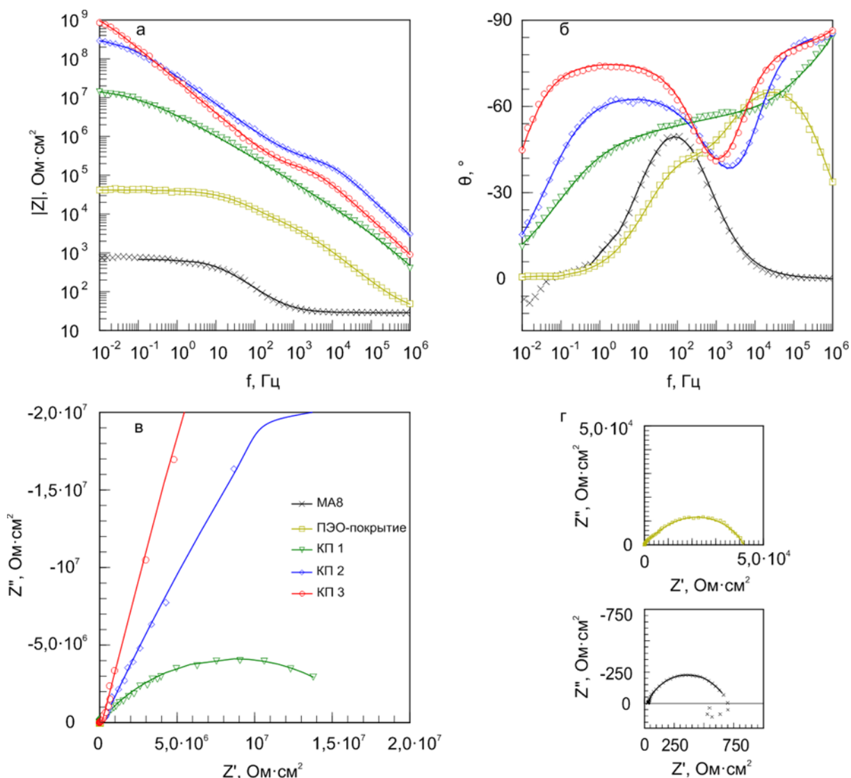
Рисунок 4.12 – Диаграммы Боде (а, б) и Найквиста (в, г) для образцов из магниевого сплава МА8 после разной поверхностной обработки. Символами обозначены экспериментальные данные, линией – теоретические кривые, рассчитанные в соответствии с предложенными ЭЭС
