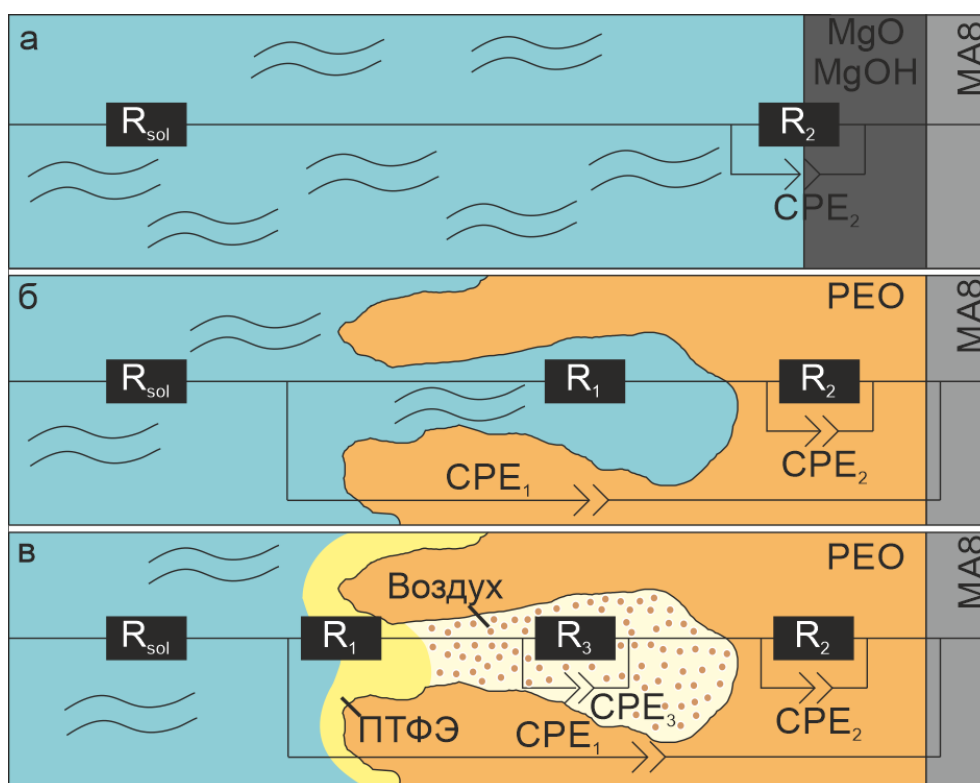
Рисунок 4.11 – Модели структуры покрытий и соответствующие эквивалентные электрические схемы, применяемые для моделирования экспериментальных импедансных данных: для магниевого сплава без покрытия (а), для ПЭО-покрытия (б) и композиционных покрытий (в) [134]
