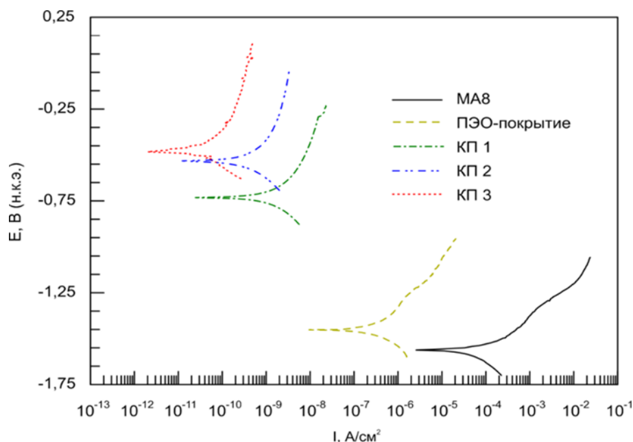
Рисунок 4.13 – Потенциодинамические поляризационные кривые образцов из магниевого сплава МА8 с разными видами поверхностной обработки
