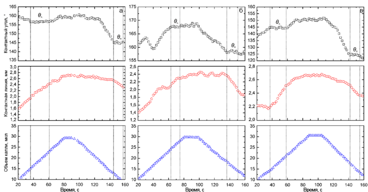
Рисунок 4.7 – Графики изменения контактного угла (верхняя панель), длины контактной линии (средняя панель) и объема капли (нижняя) в процессе измерения углов натекания и оттекания на поверхности КП 1 (а), КП 2 (б) и КП 3 (в), сформированных на магниевом сплаве МА8
