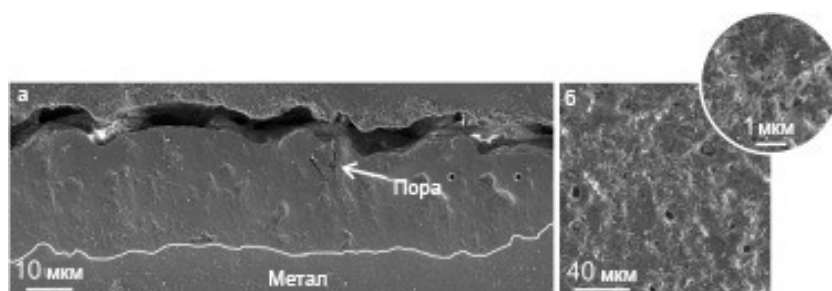
Рисунок 4.5 – СЭМ-изображения поперечного сечения (а) и поверхности (б) модифицированного композиционного покрытия [164]
