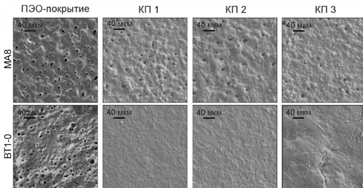
Рисунок 4.3 – СЭМ-изображения поверхности ПЭО- и композиционных покрытий на магниевом сплаве и титане марки BT1-0
