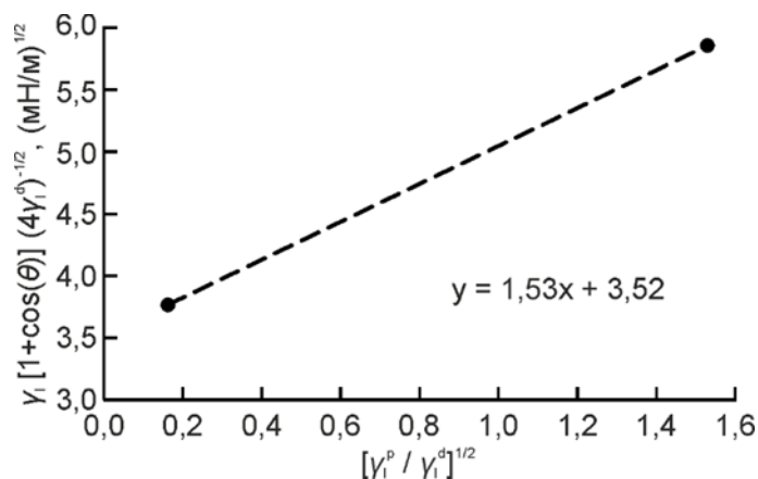
Рисунок 2.2. График линейаризованного уравнения Оуэнса (модель ОВРК) для ПТФЭ ( R_a = 0,5 мкм)
