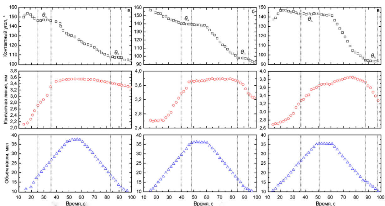
Рисунок 4.8 – Графики изменения контактного угла (верхняя панель), длины контактной линии (средняя) и объема капли (нижняя) в процессе измерения углов натекания и оттекания на поверхности КП 1 (а), КП 2 (б) и КП 3 (в), сформированных на титане марки VT1-0 [161]
