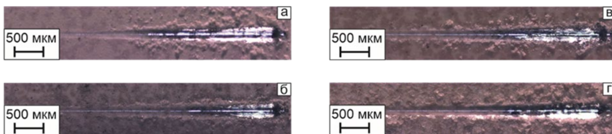
Рисунок 4.17 – Оптические изображения царапин, нанесенных на поверхность ПЭО-покрытия (а) и композиционных покрытий КП 1 (б), КП 2 (в), КП 3 (г), полученных на магниевом сплаве МА8
