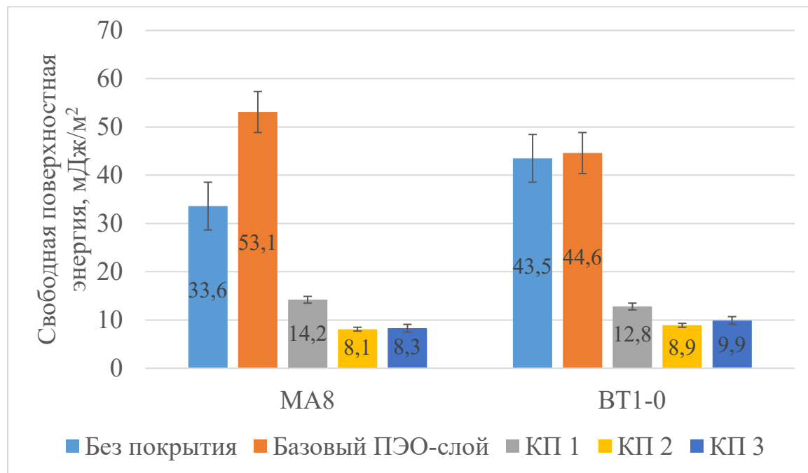
Рисунок 4.9 – Расчетные значения свободной поверхностной энергии исследуемых образцов
