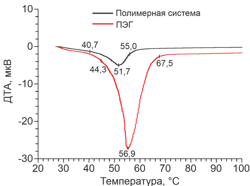
Рисунок 3.3 – Дифференциальный термический анализ полимерной системы и исходного полиэтиленгликоля
