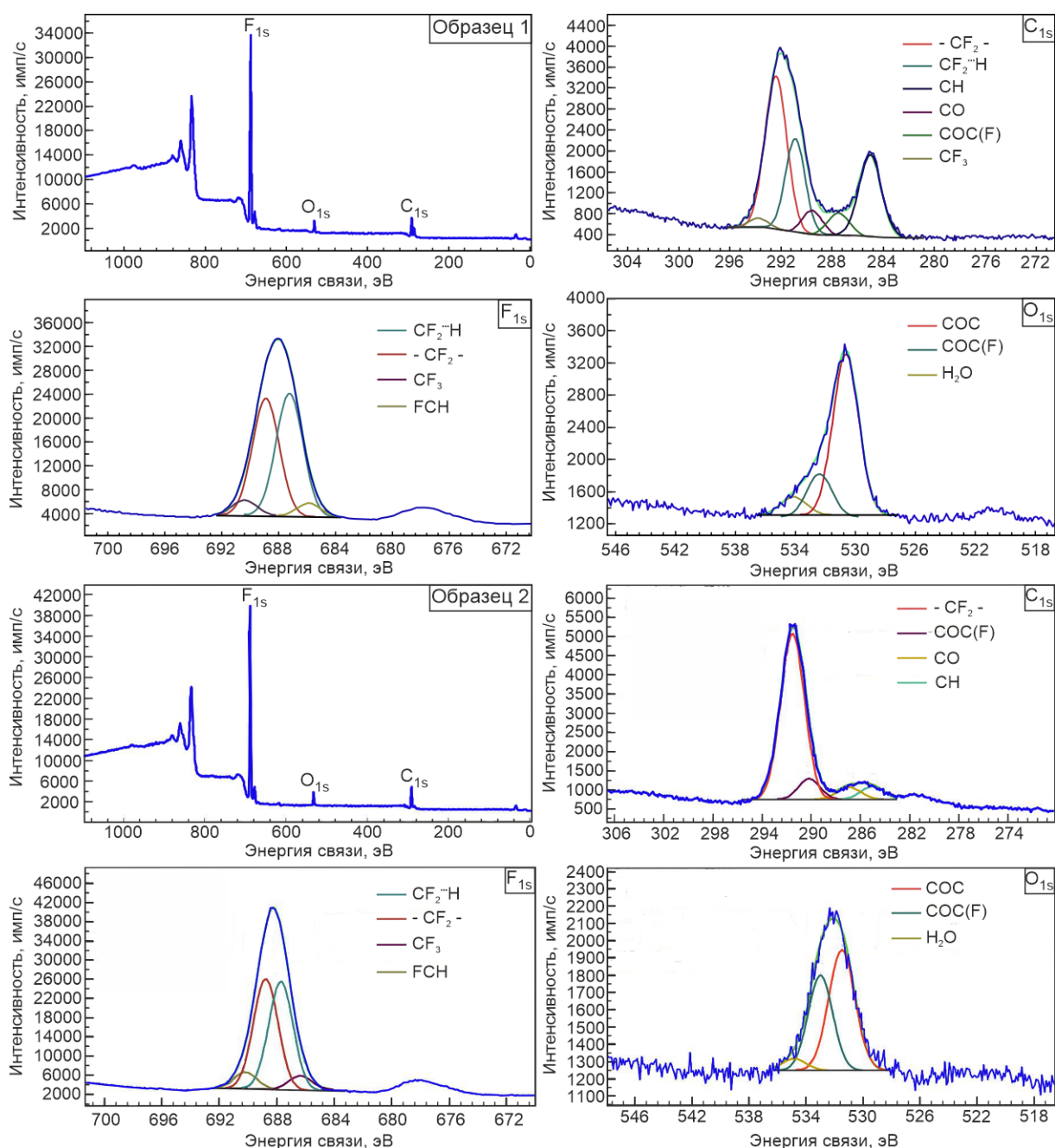
Рисунок 3.5 – Обзорный спектр и спектры высокого разрешения для образцов 1 и 2 с разложением основных пиков элементов полимерной системы.
