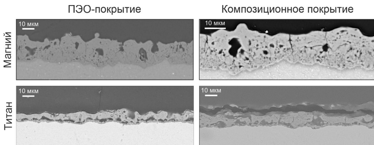
Рисунок 4.2 – СЭМ-изображения поперечного шлифа ПЭО-покрытий и КП 2 на магниевом сплаве и титане BT1-0
