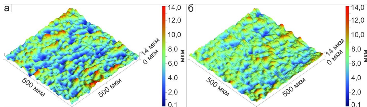
Рисунок 3.8 – 3D-профили поверхности базового ПЭО-слоя (а) и композиционного слоя с нанесением полимерной системы на поверхность базового ПЭО-слоя (б)
