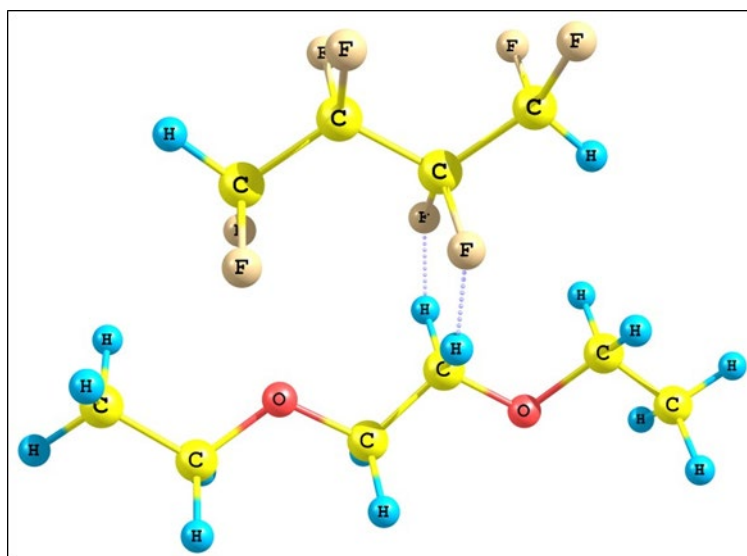
Рисунок 3.7 – Модель октофторбутана и диэтилового эфира этиленгликоля для расчета энергии нековалентных связей фтор–водород
