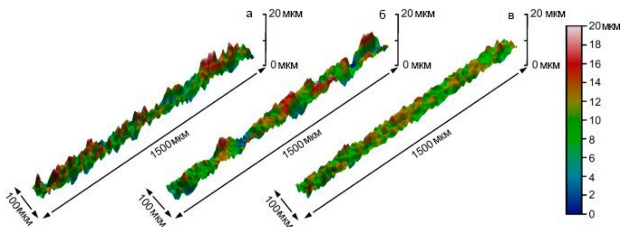
Рисунок 4.6 – 3D-профили поверхности ПЭО-покрытия (а), композиционного покрытия, полученного путем погружения в УПТФЭ (б), и МКП, полученного путем погружения в УПТФЭ с последующим распылением раствора теломеров (в) [164]
