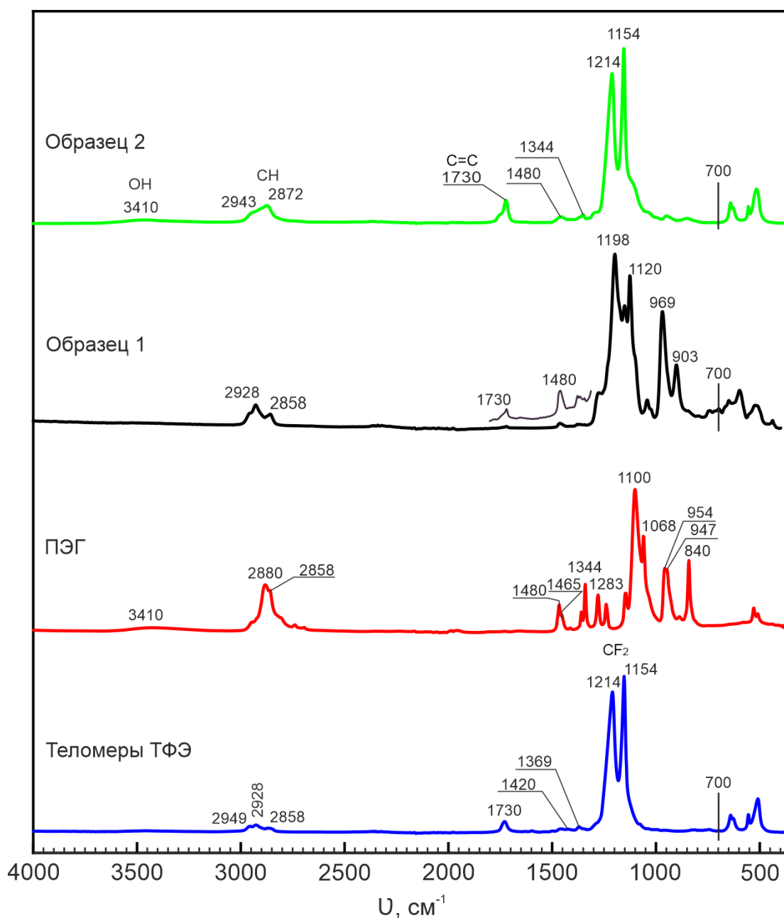
Рисунок 3.4 – ИК-спектры пленок, полученных из растворов теломеров ТФЭ в ацетоне (синий), полиэтиленгликоля (красный), полимерной системы ПЭГ -теломеры ТФЭ: Образец 1 (черный) и Образец 2 (зеленый)
