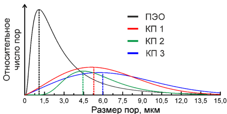
Рисунок 4.4 – Распределение пор по размерам для ПЭО- и композиционных покрытий на магниевом сплаве МА8
