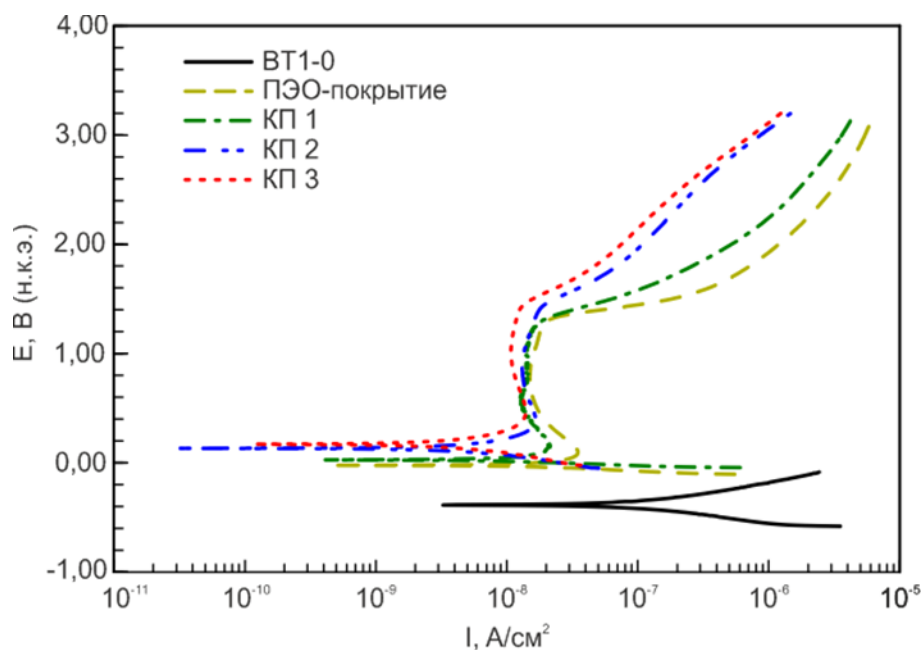
Рисунок 4.15 – Потенциодинамические поляризационные кривые образцов из технически чистого титана марки ВТ1-0 с разными видами поверхностной обработки [165]
