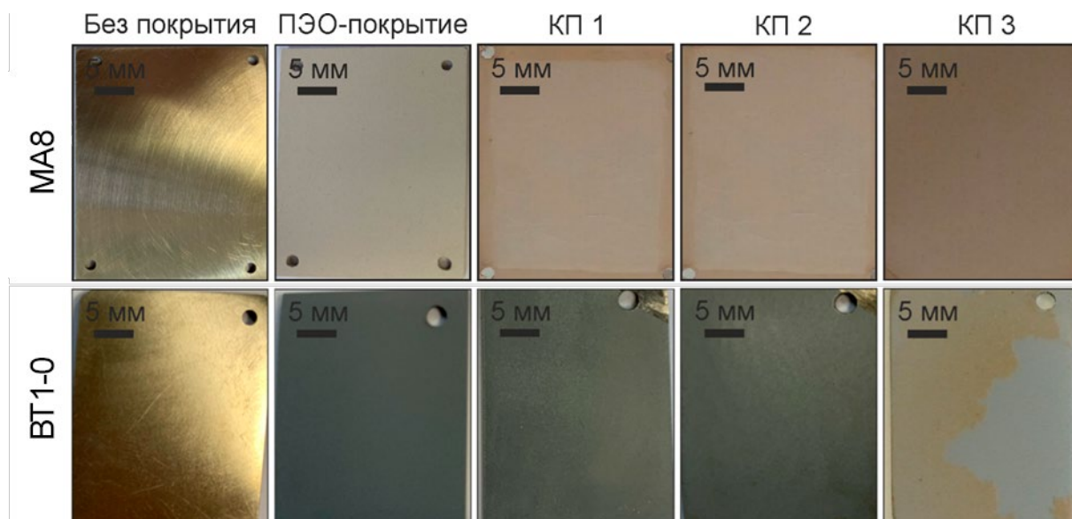
Рисунок 4.1. – Оптические изображения материалов без покрытия, с ПЭО-покрытием и композиционными покрытиями КП 1, КП 2 и КП 3
