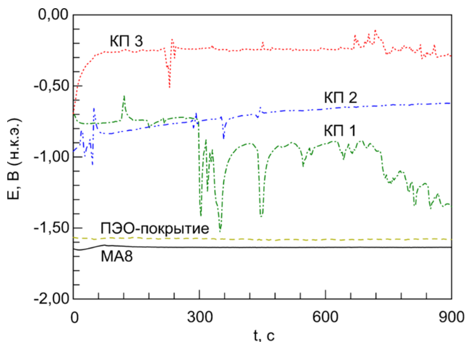
Рисунок 4.10 – Динамика изменения электродного потенциала в течение 15 мин выдержки в 3,5 масс.% растворе NaCl для образцов с разными видами поверхностной обработки
