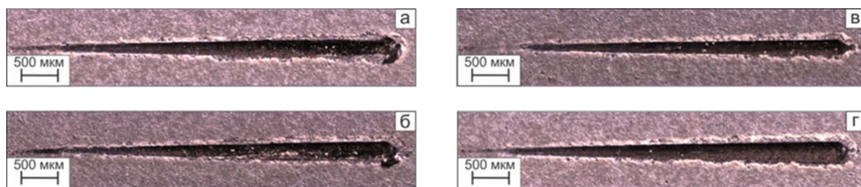
Рисунок 4.18 – Оптические изображения царапин, нанесенных на поверхность ПЭО-покрытия (а) и композиционных покрытий: КП 1 (б), КП 2 (в), КП 3 (г), полученных на титане марки ВТ1-0
