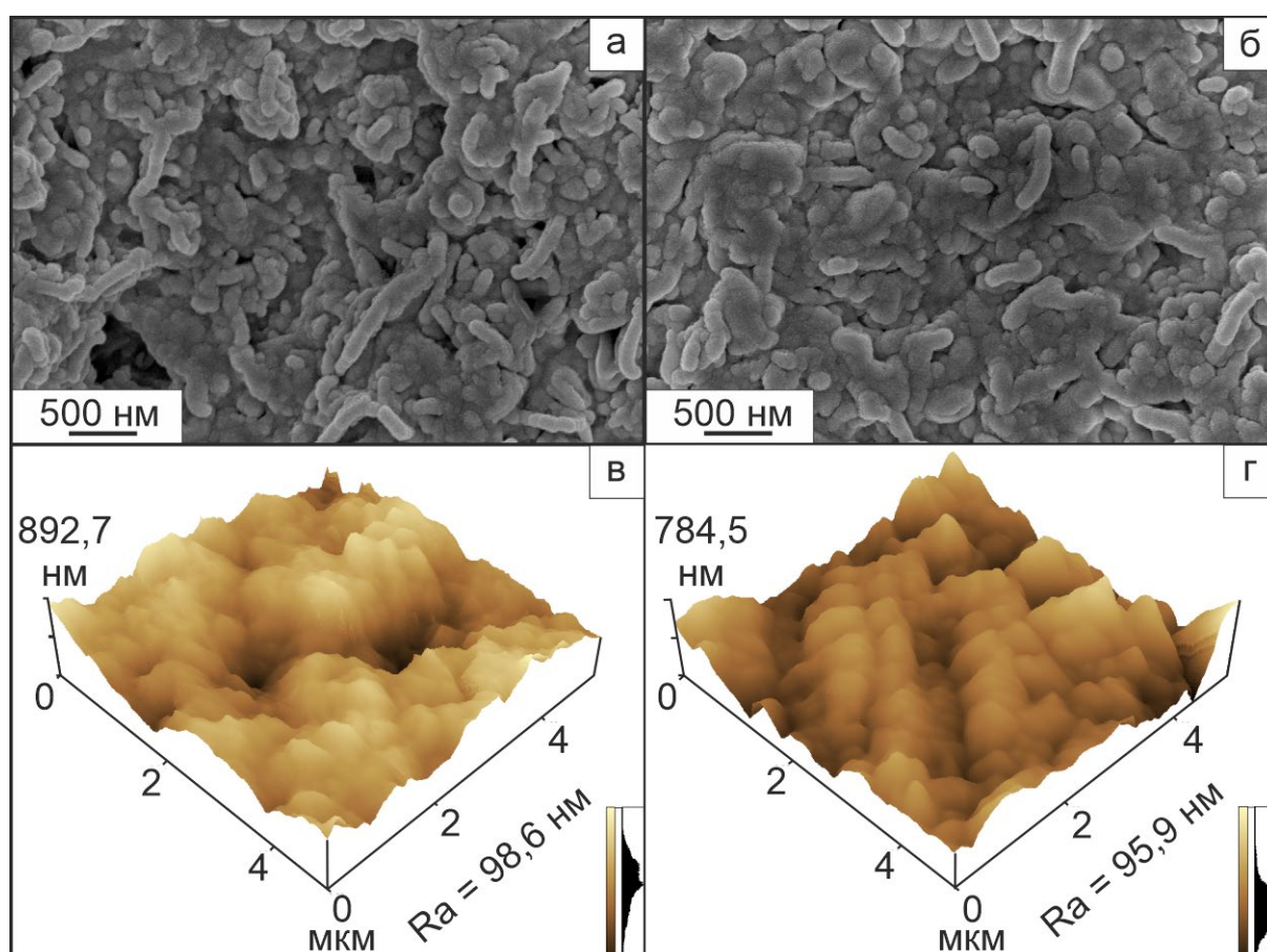
Рисунок 3.2 – Морфология пленки полимерной системы до (а, в) и после термической активации (б, г). Показаны изменения, фиксируемые СЭМ (а, б) и АСМ (в, г)
