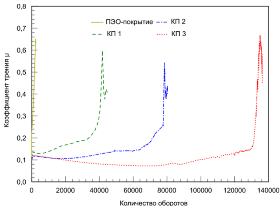
Рисунок 4.16 – Зависимость коэффициента трения от количества циклов для образцов из магниевового сплава МА8 без покрытия, с ПЭО-покрытием и с композиционными покрытиями
