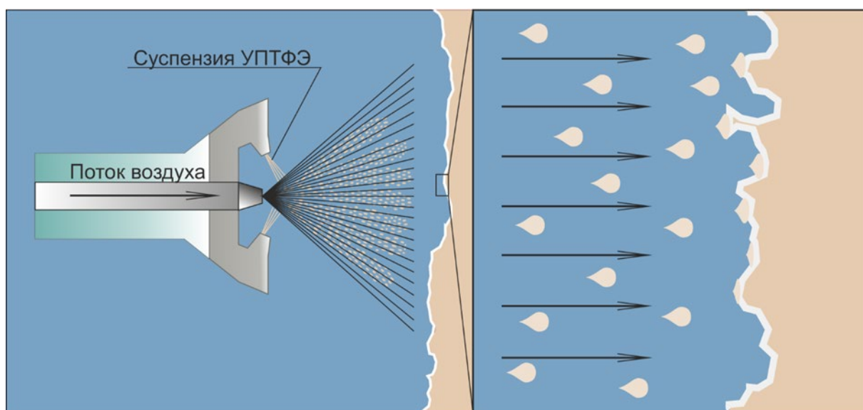
Рисунок 2.1. – Схема нанесения ультрадисперсного политетрафторэтилена методом распыления
